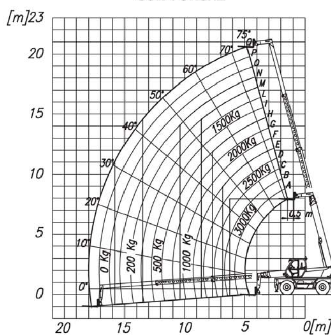
FRONTALE SU GOMME CON FORCHE
